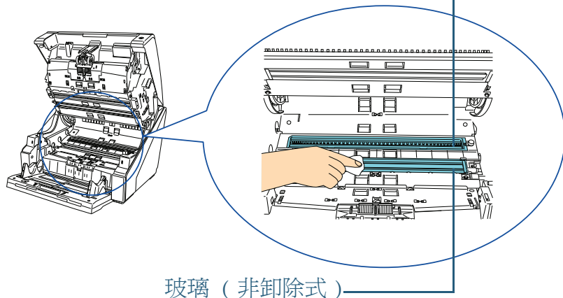
玻璃（卸除式）
