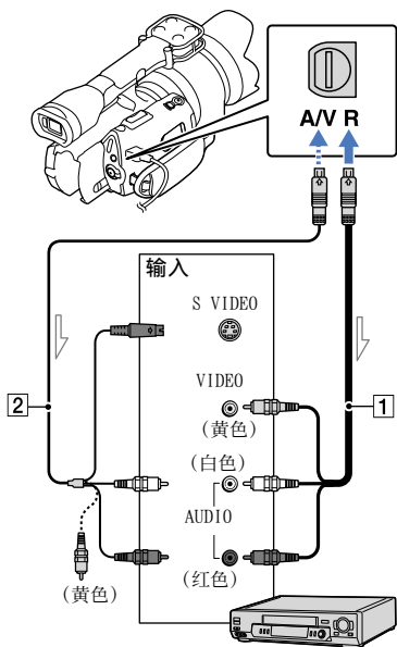
— 信号流
