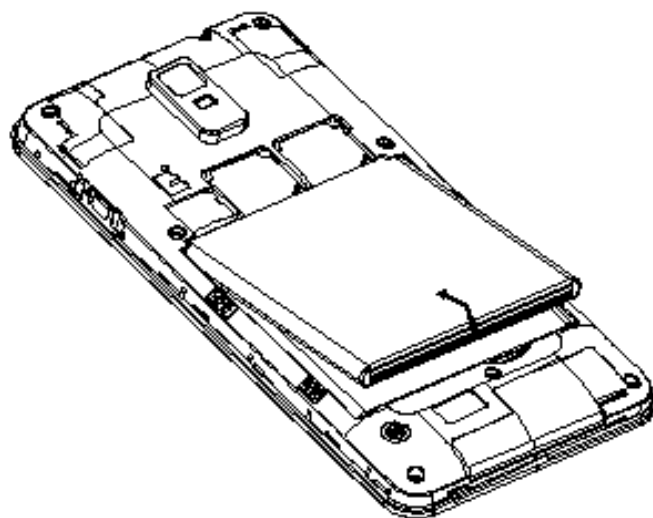
电池拆卸图2
