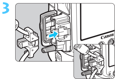
线夹
