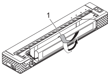
1 电池取出带
