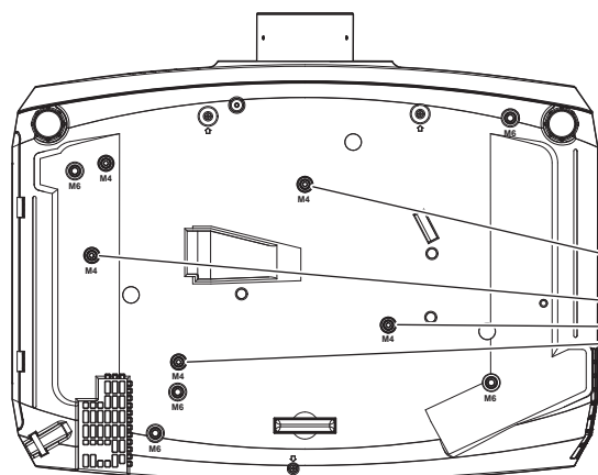
底部视图
