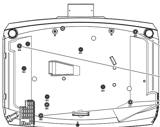
底部视图
