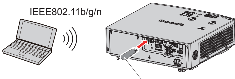
选配件无线传输模块（型号：AJ-WM50MC）
