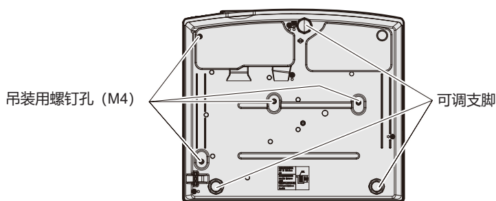
吊装用螺钉孔位置和可调支脚
