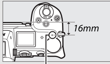
焦平面标记
