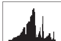
▲ 曝光良好
