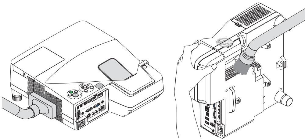
抽吸散热孔中的灰尘。
