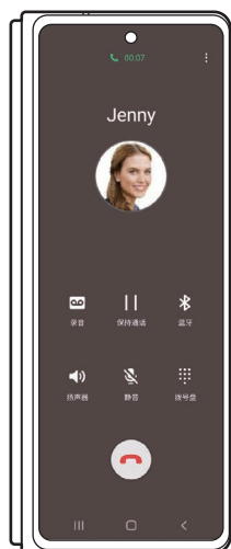
电话
