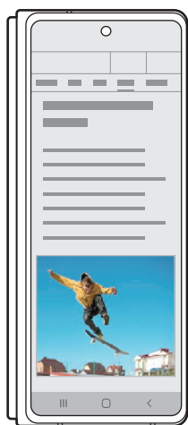
外屏
