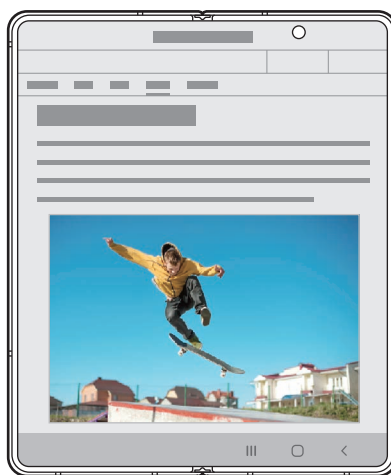
主屏幕
