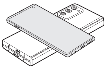
智能手机
