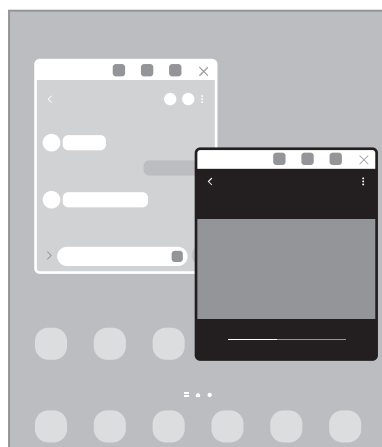
弹出视图
