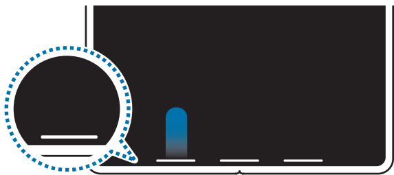
从底部滑动
