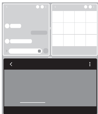
分屏视图
