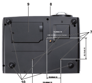
底部概览
