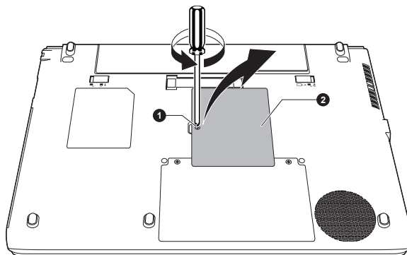
圖 4-11 移除記憶體模組蓋板(R940)
