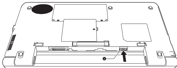
圖 4-8 移除 SIM 卡(R940)
