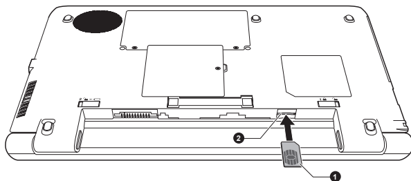
圖 4-7 安裝 SIM 卡(R940)
