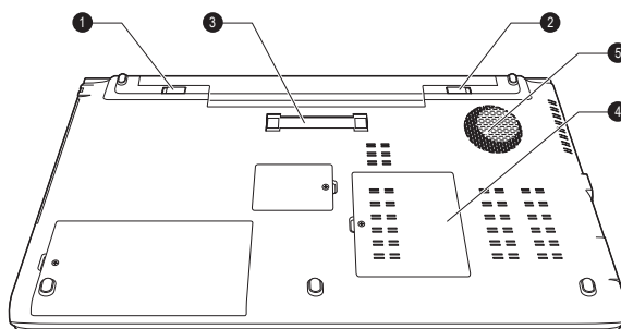
圖 3-5 電腦底部(R950)
