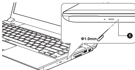
圖 4-6 使用彈出孔手動彈出托架(R940)
