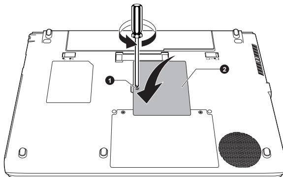
圖 4-13 蓋上記憶體模組蓋板(R940)
