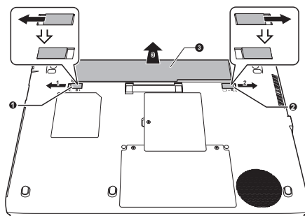
圖 4-10 釋放電池組(R940)
