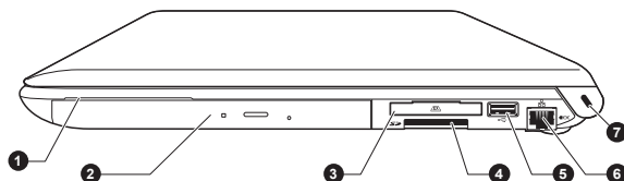
圖 3-9 電腦右側(R940)
