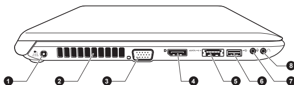
圖 3-8 電腦左側(R940)
