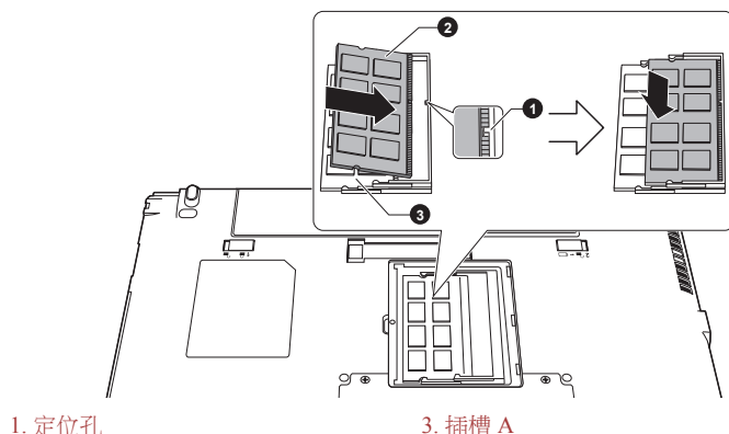
圖 4-12 安裝記憶體模組 (R940)
