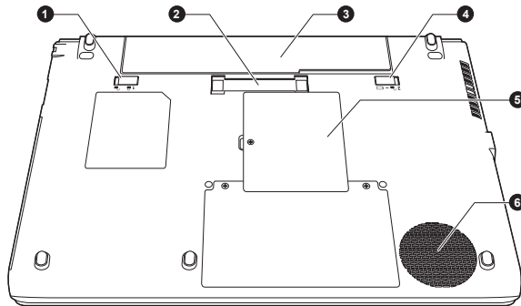
圖 3-11 電腦底部(R940)
