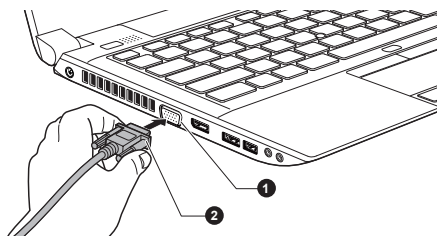
圖 4-18 將顯示器纜線連接到外接 RGB 顯示器埠(R940)
