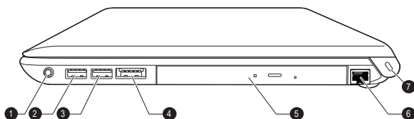
圖 3-3 電腦右側(R950)
