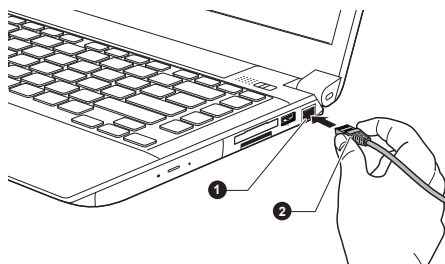
圖 4-9 連接 LAN 纜線(R940)
