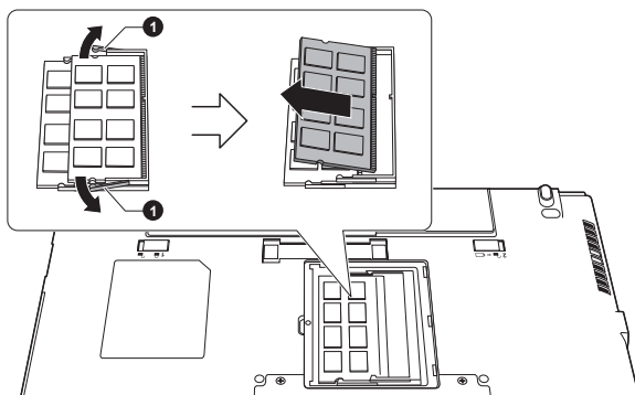
圖 4-14 移除記憶體模組(R940)
