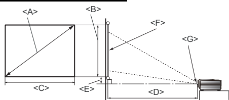
桌上安装
