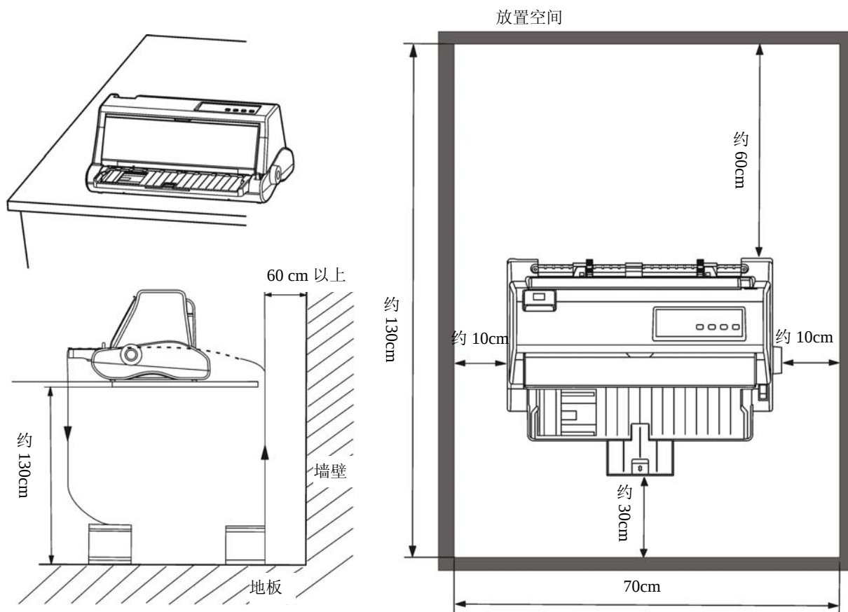
图 2-5 打印机放置
