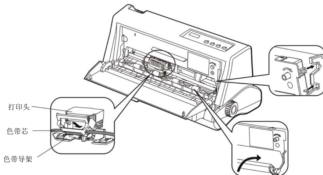
图 2-9 安装色带盒
