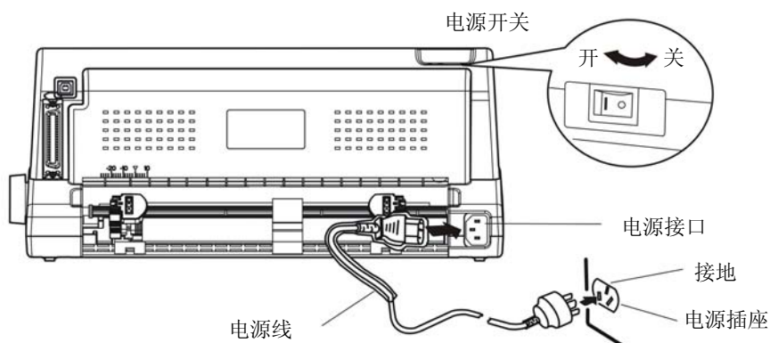
图 2-10 连接电源线
