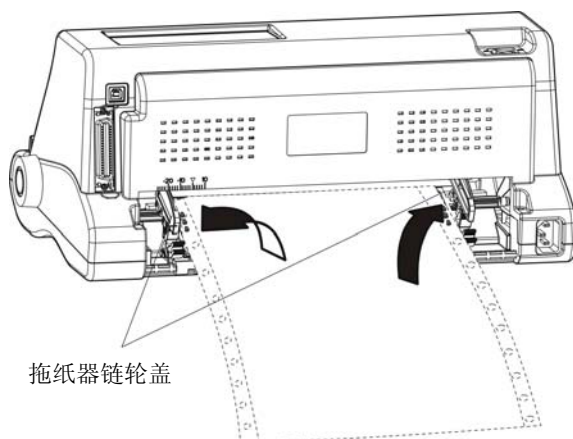
图 3-11 将连续纸安装在拖纸器上
