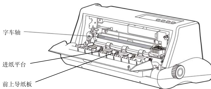
图 A-1 清洁打印机
