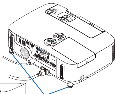
背部支脚
