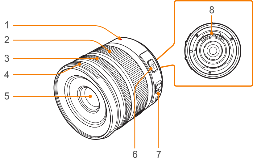
SAMSUNG 18-55 mm F3.5-5.6 OIS II 镜头（示例）
