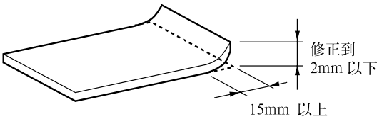
弯曲
