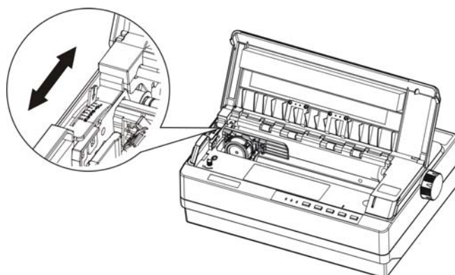
图 2-3 纸厚调节杆
