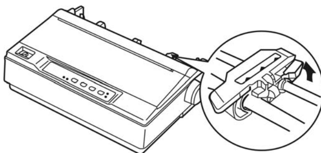
图 3-7 松开链轮
