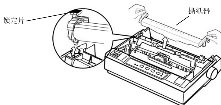
图 1-16 卸下撕纸器
