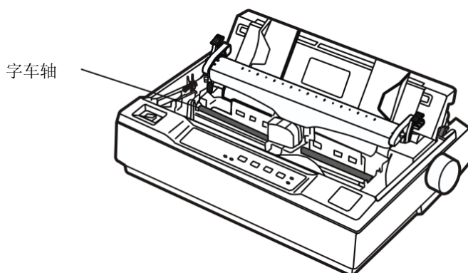
图 5-1 清洁打印机
