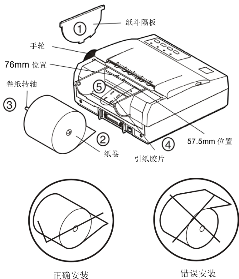
图 3-7 纸卷安装
