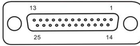
图 D-6 串行接口插座引脚序号
