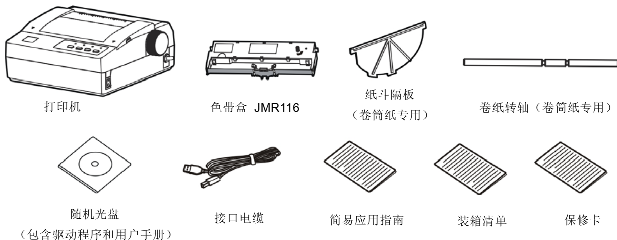
图 1-1 打印机包装箱内组件
