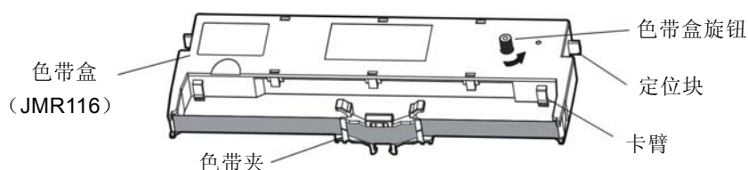
图 1-6 色带盒
