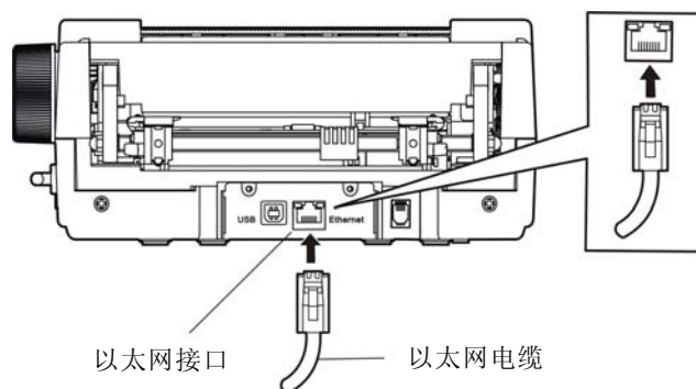
图 1-13 连接以太网电缆
