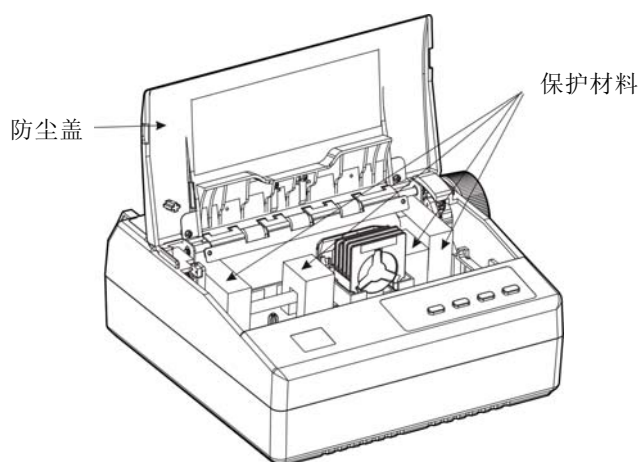
图 1-2 拆除保护材料
