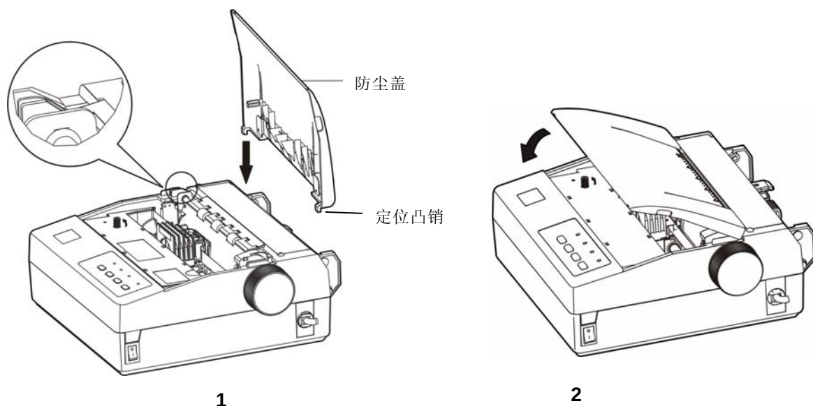
图 1-8 安装防尘盖
