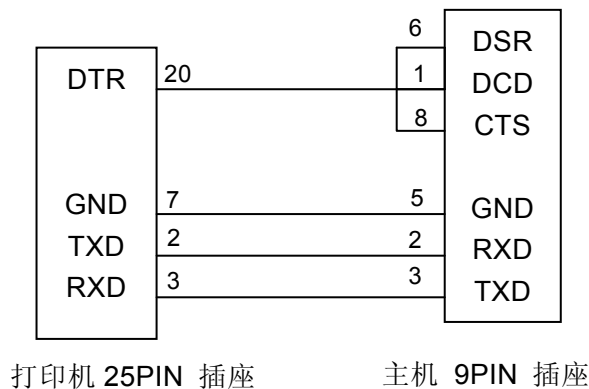
图 D-7 主机与打印机的连接示意图
