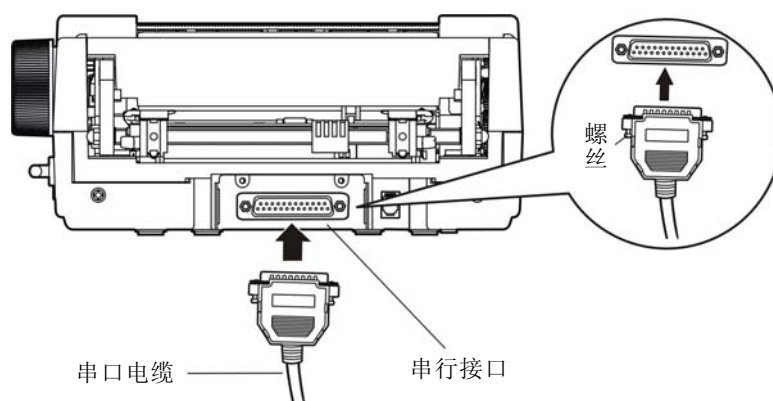
图 1-12 连接串口电缆
