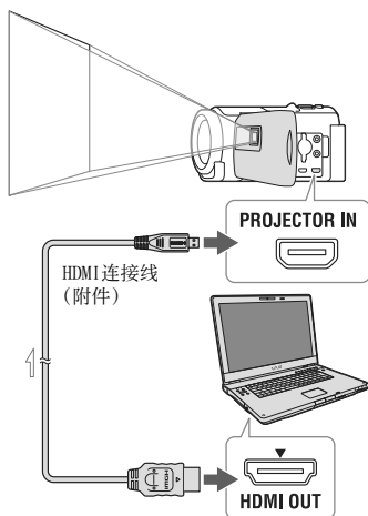
信号的流向
