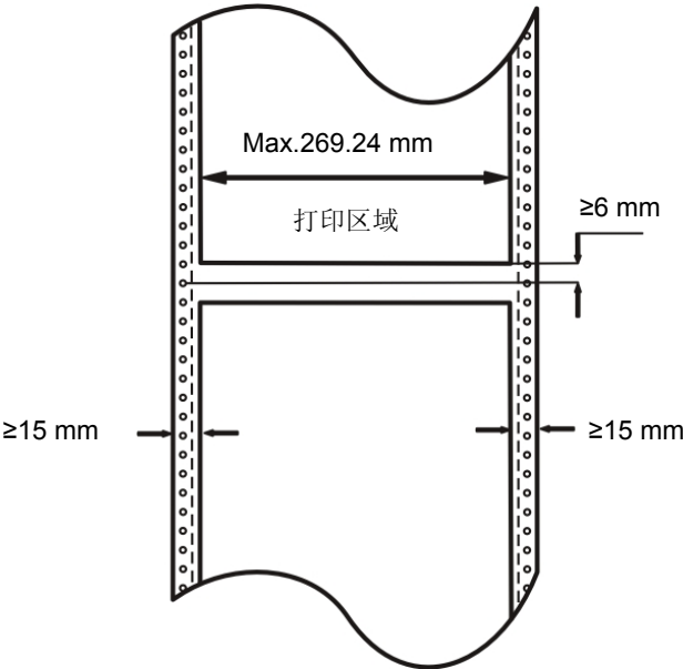
图 B-8 连续纸打印区域
