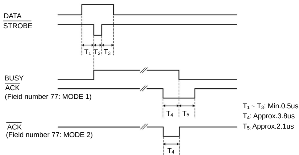
图 B-1 时序图
