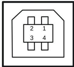
图 B-3 USB-B 型插座
