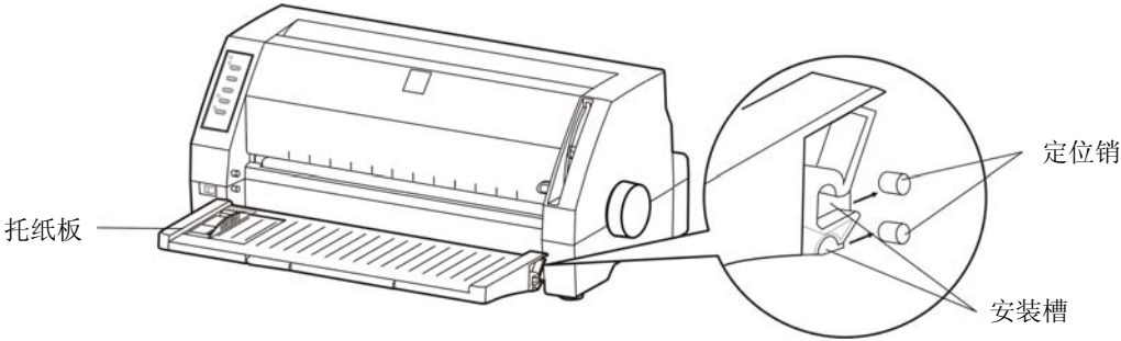
图 2-5 安装托纸板
