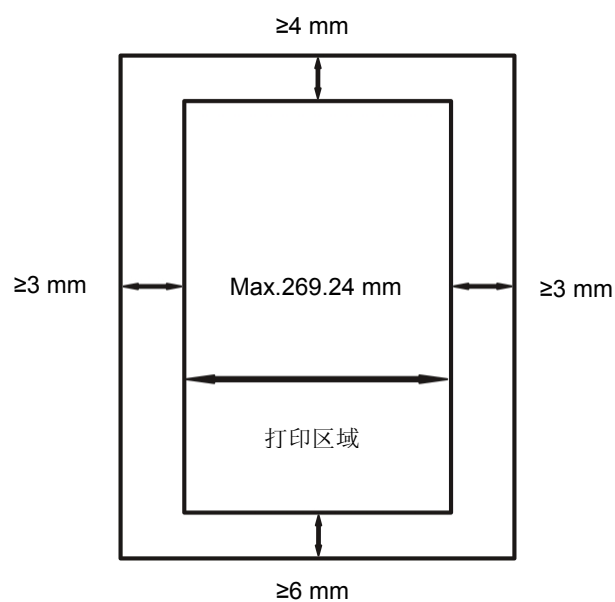
图 B-7 单页纸打印区域
