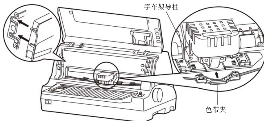
图 2-10 安装色带盒
