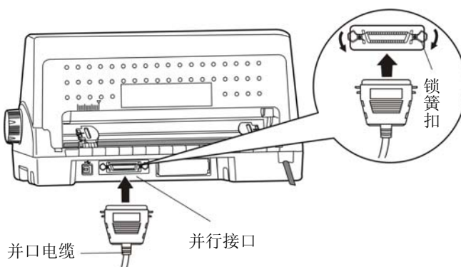
图 2-12 连接并行接口电缆
