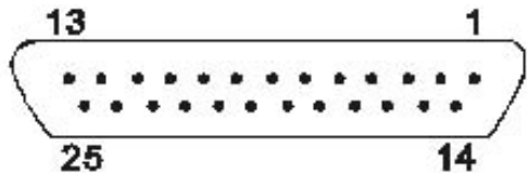
图 B-4 并行接口插座引脚序号
