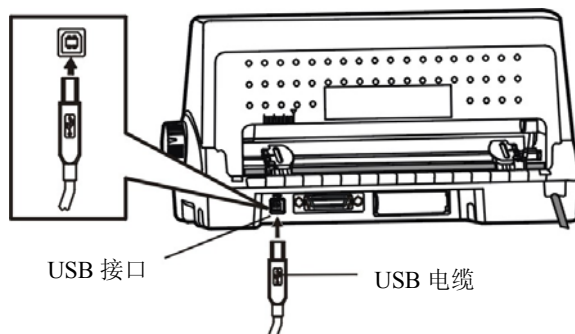
图 2-11 连接 USB 电缆
