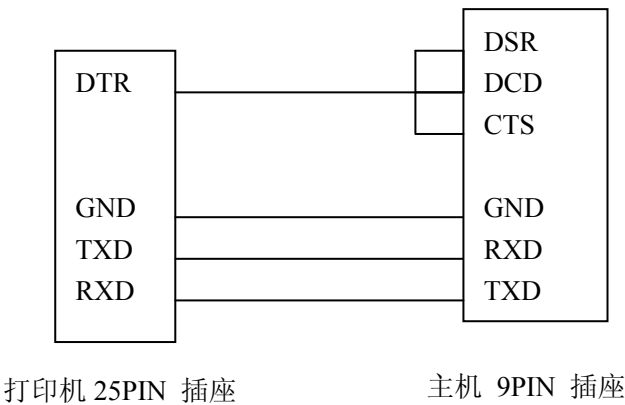
图 B-6 打印机与主机的连接
