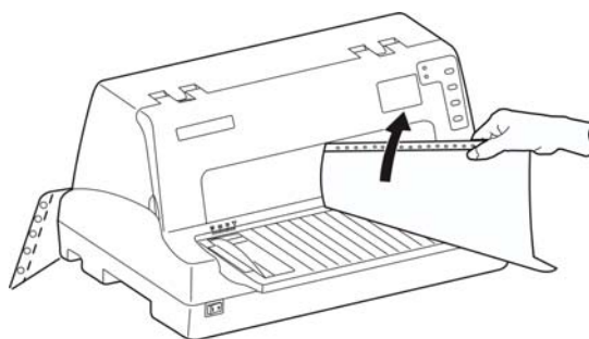
图 3-11 撕连续纸
