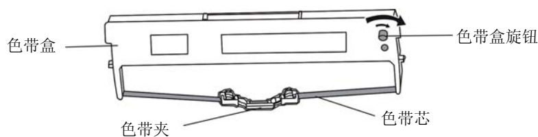
图 2-9 色带盒
