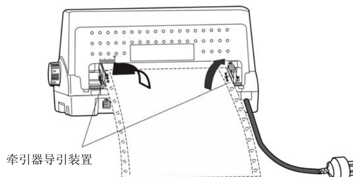
图 3-8 将连续纸安装在牵引器上
