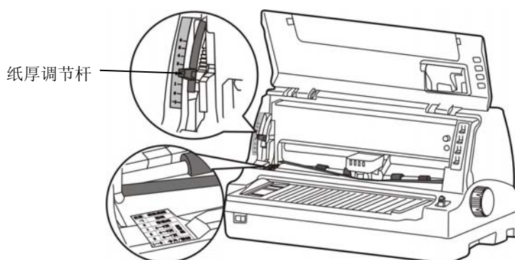
图 3-1 调整纸厚调节杆
