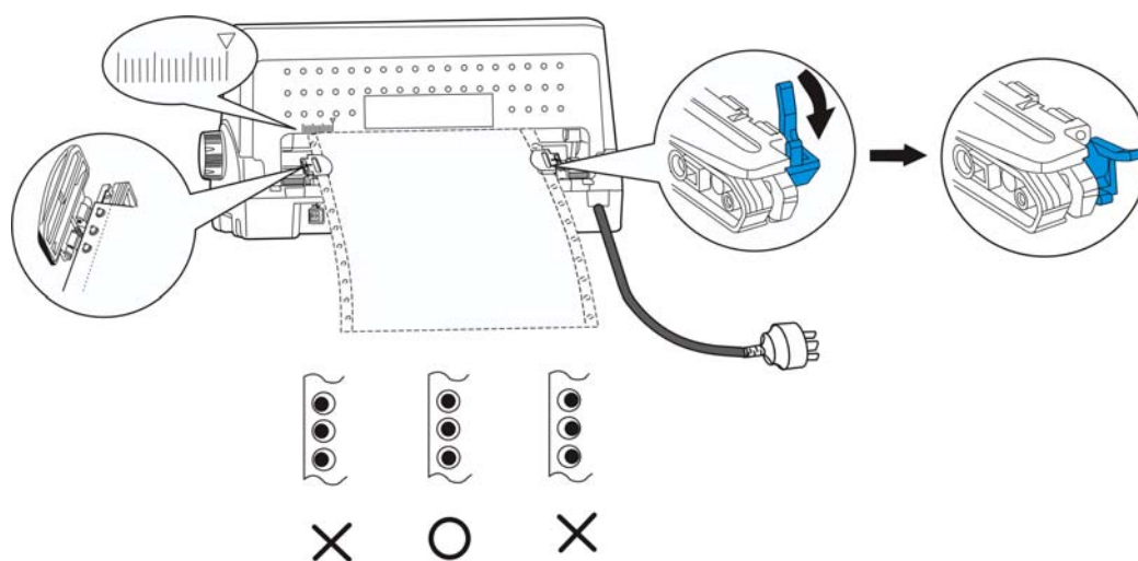
图 3-10 调整右边牵引器位置
