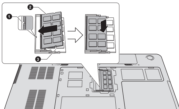
圖 3-14 蓋上記憶體模組
