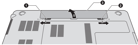
圖 5-2 釋放電池組-2
