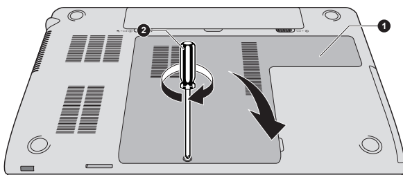
圖 3-15 蓋上記憶體模組蓋板
