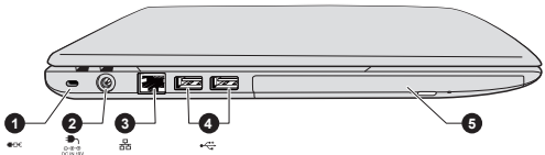
圖 2-2 電腦左側
