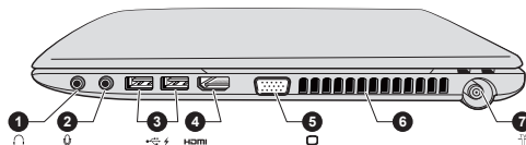
圖 2-3 電腦右側
