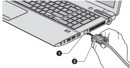
圖 3-18 將顯示器纜線連接到外接 RGB 顯示器埠。
