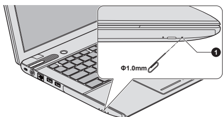
圖 3-8 使用彈出孔手動彈出托架
