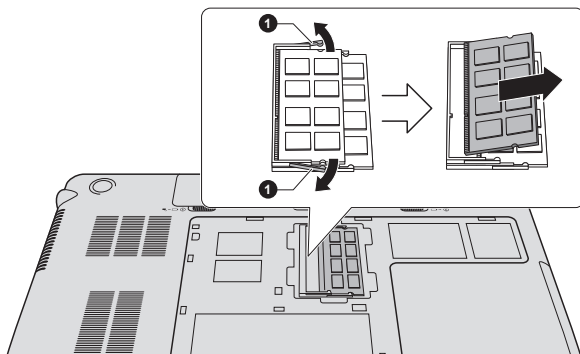
圖 3-16 移除記憶體模組
