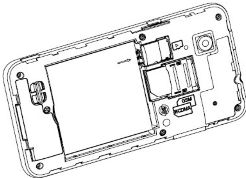
图 1 存储卡插入
