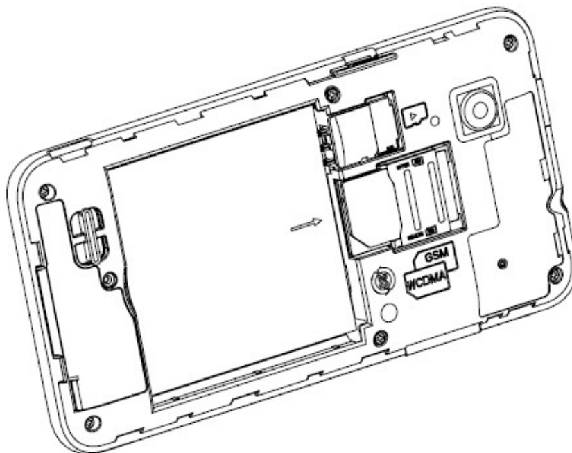
图1 SIM卡插入
