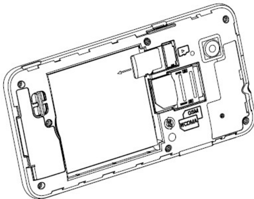
图 2 存储卡取出
