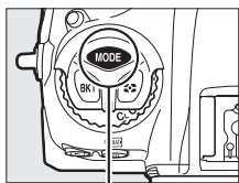
MODE 按钮
