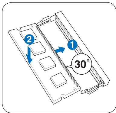
安装内存条
