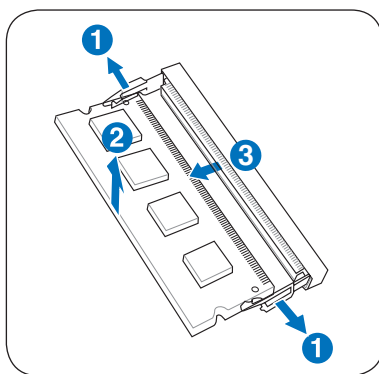
移除内存条
