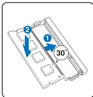
安装内存条
