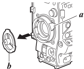
a. 镜头固定杆 b. 接口盖
